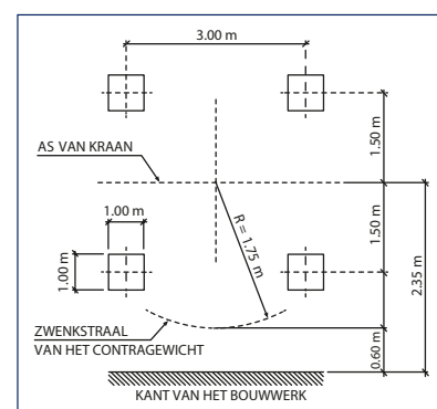
GRONDOPPERVLAK
